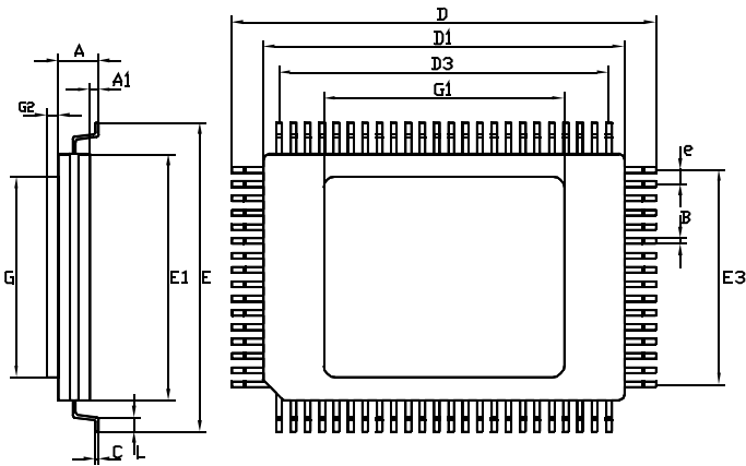
CQFP080
